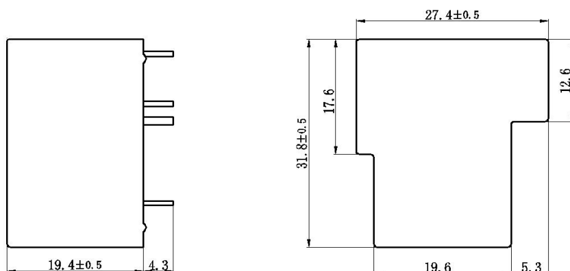
外型图 OUTLINE
