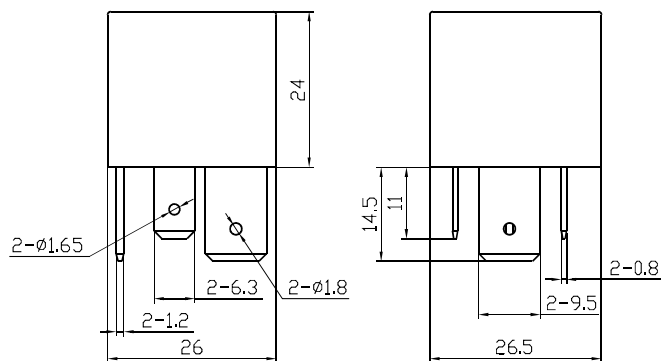
长脚型 Long foot
