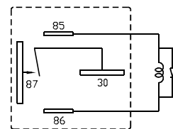
带二极管型 With diode
