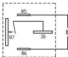
普通型 Without accessory
