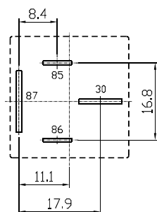
安装孔位图 (底视图) PCB Layout ( Bottom View )
