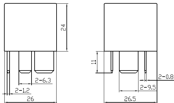
短脚型 Short foot
