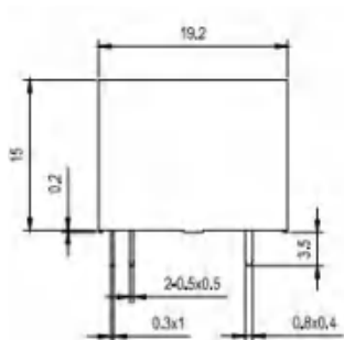
外形尺寸图
