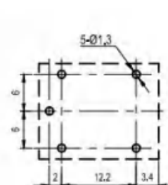
安装尺寸图
