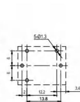
安装尺寸图
