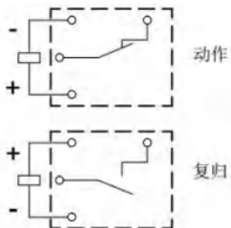
接线图
