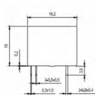
外形尺寸图
