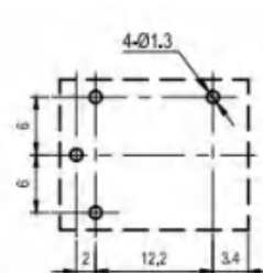
安装尺寸图
