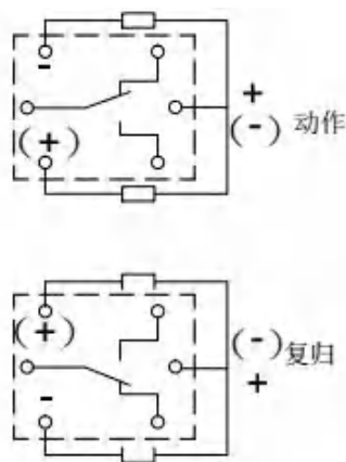
接线图
