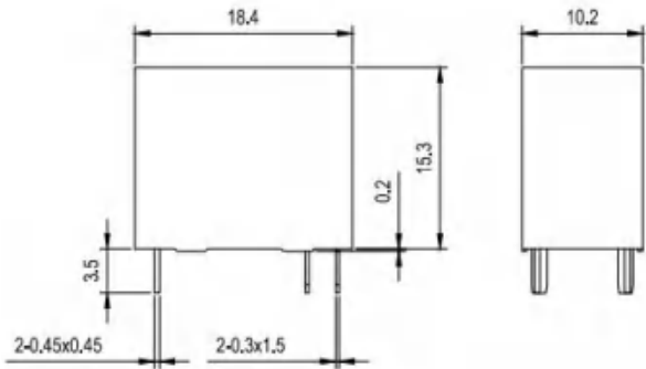
外形尺寸图
