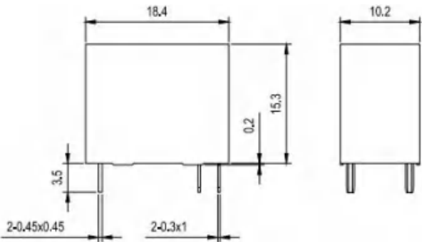
外形尺寸图
