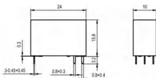
1A/1B(双线圈)
