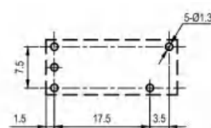
(底视图)
