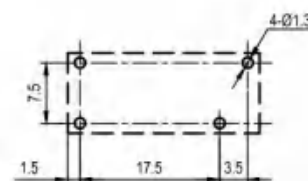
(底视图)
