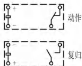
接线图
