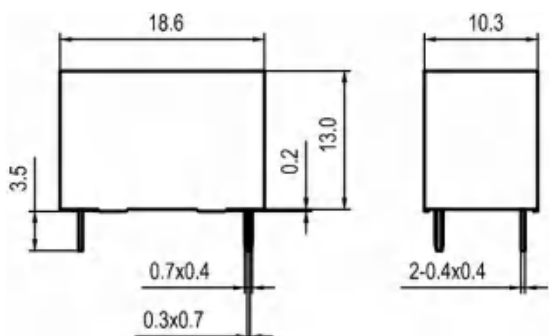
外形尺寸图
