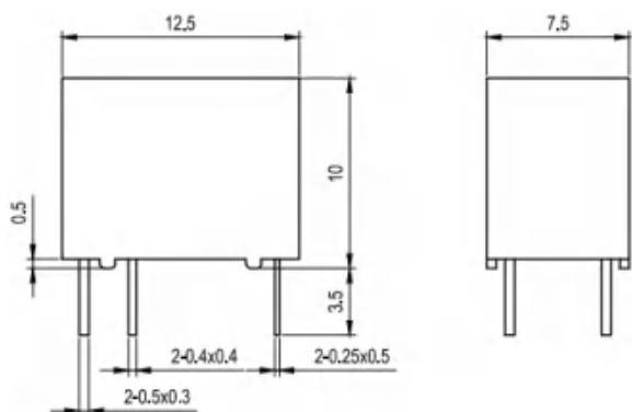
外形尺寸图
