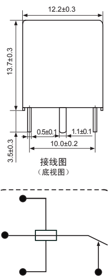
外形图
