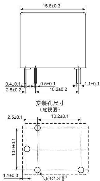
外形图
