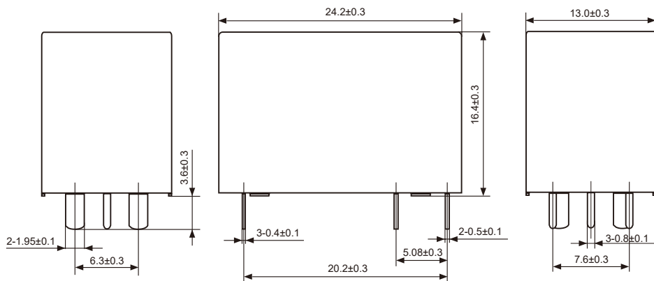
外形图
