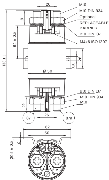
Change-over NO/NC
